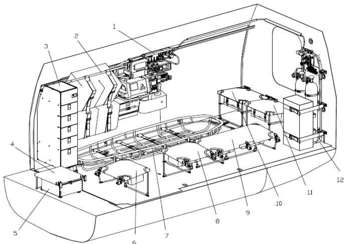
Rys. 6-33. Wyposażenie medyczno - ratownicze kabiny ładunkowej w wariantcie ratowniczym
