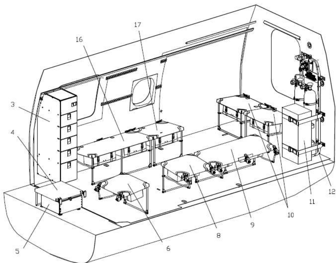
Rys 6-36 Wyposażenie medyczno - ratownicze kabiny ładunkowej w wariantcie transportowym
