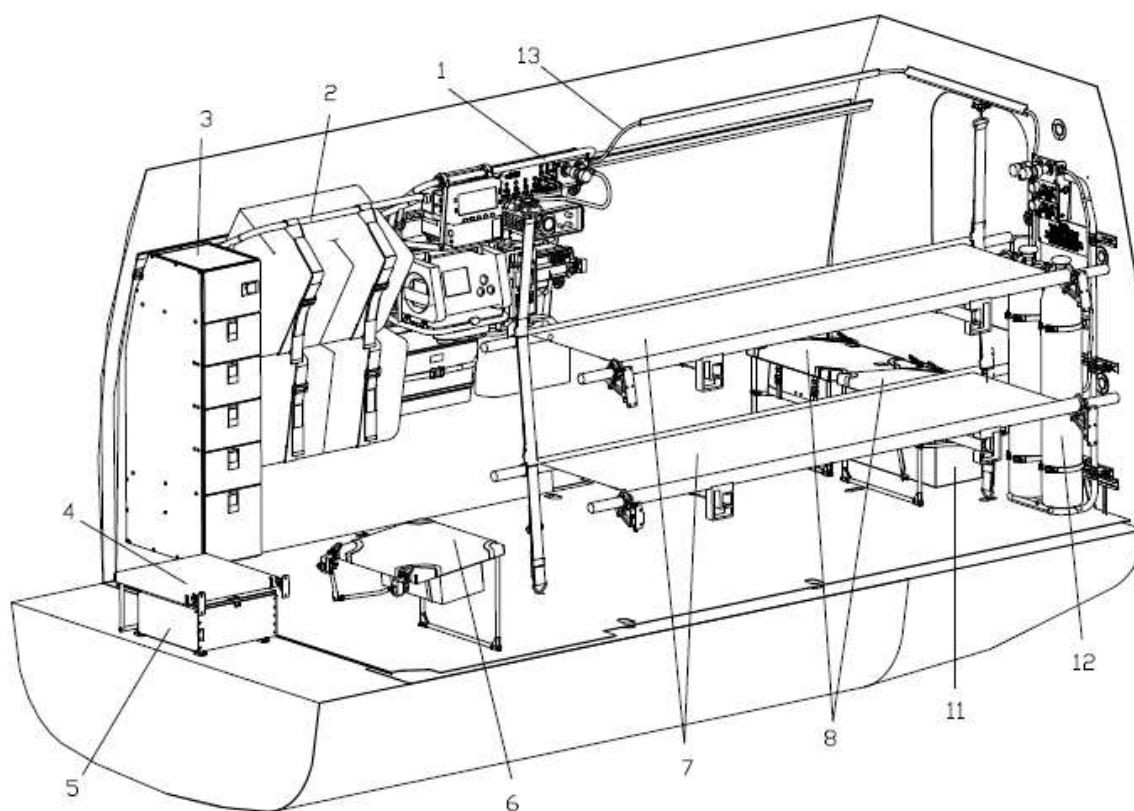
Rys 6-35 Wyposażenie medyczno - ratownicze kabiny ładunkowej w wariantcie wielonoszowym
