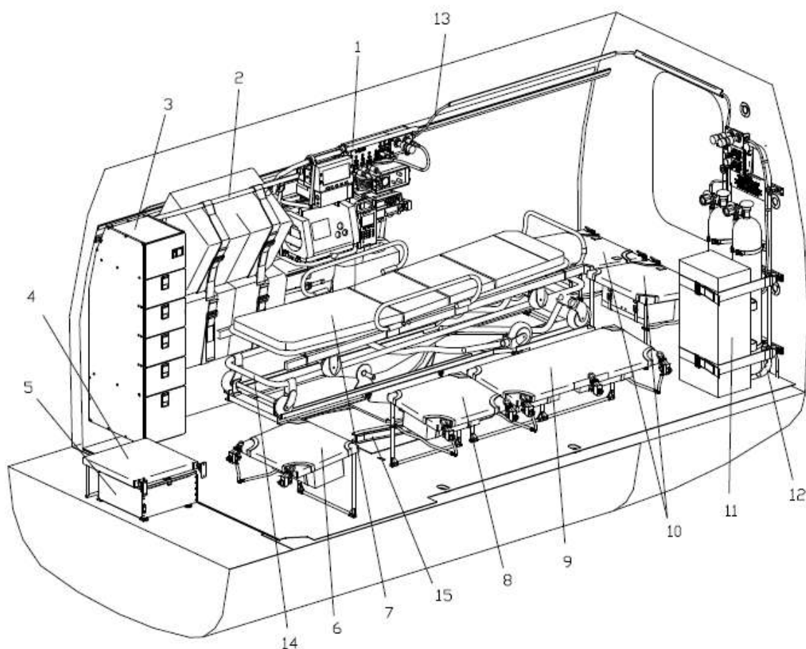
Rys. 6-34. Wyposażenie medyczno - ratownicze kabiny ładunkowej w wariantcie reanimacyjnym
