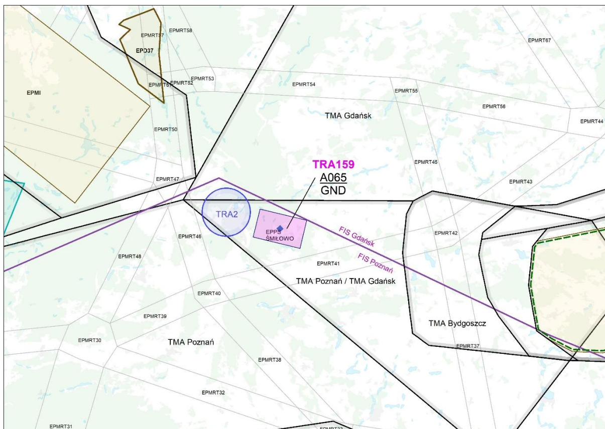
Rys 2. Planowana strefa TRA159 w rejonie lądowiska EPPS.
